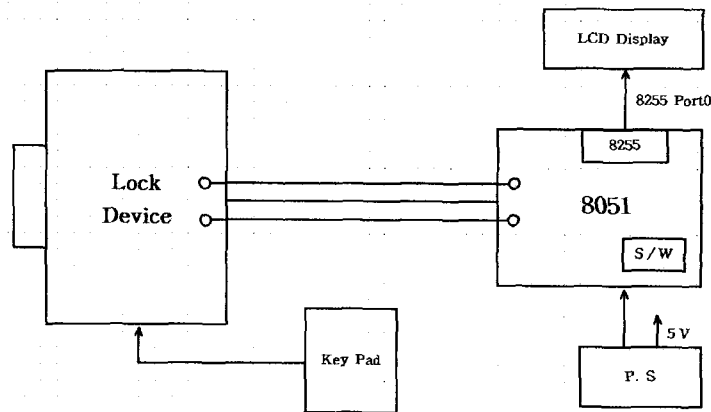
그림 13. Lock장치와 8051 제어기간 연결 구성도
