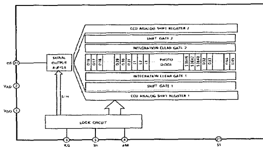
그림 3. CCD 센서 구성도 (TOSHIBA 사 TCD1305)
