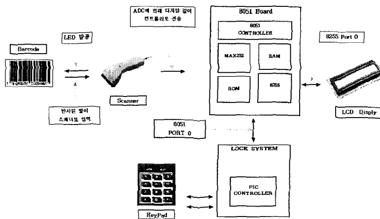
그림 12. Lock 제어를 위한 바코드 스캐너 구성도
