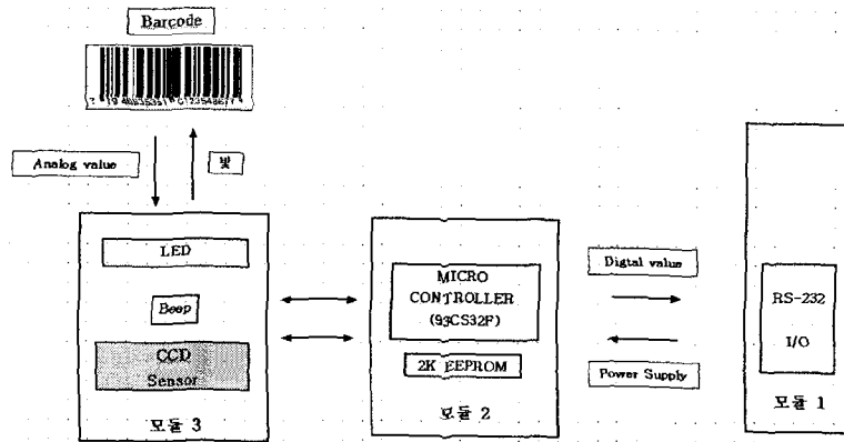
그림 11. 스캐너 모듈별 시제품 구성도
