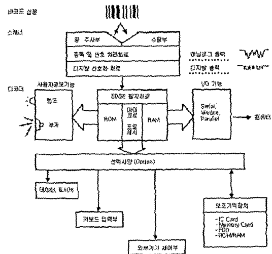
그림 2. 일반적인 바코드 스캐너 구성도
