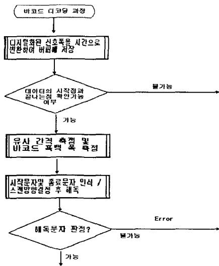
그림 9. 디코딩 소프트웨어 알고리즘
