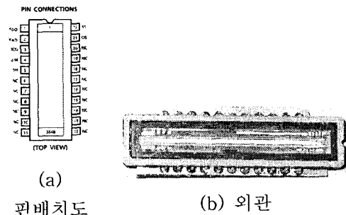
그림 4. TCD1305의 핀배치도 및 외관
