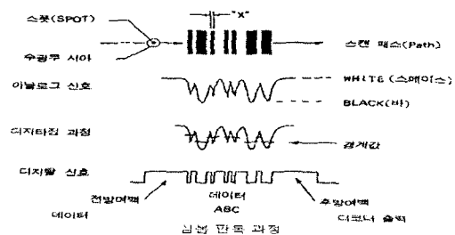
그림 8. 바코드 디지털화 과정
