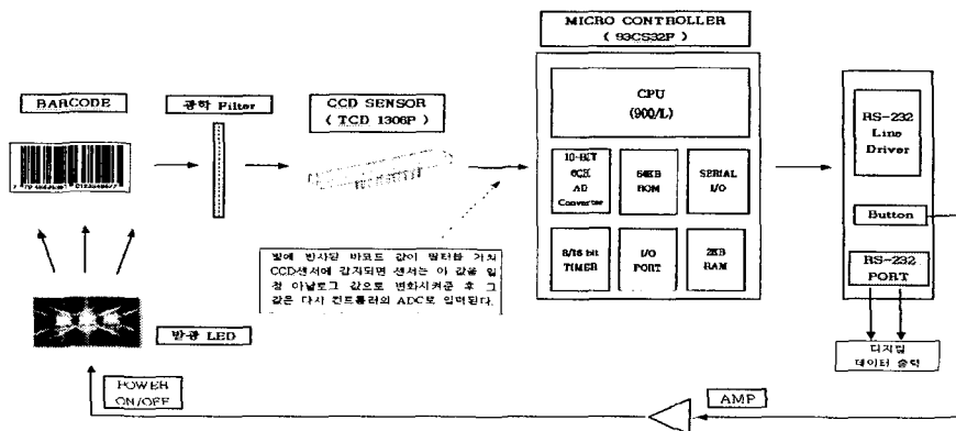
그림 10. 휴대폰 바코드 스캐너 블럭도
