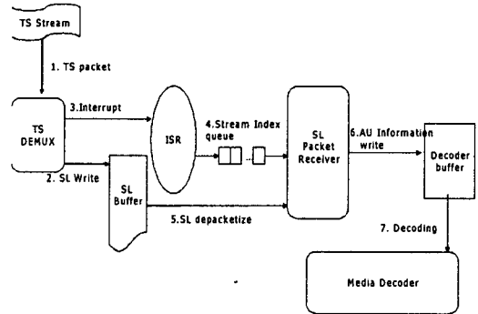
[그림 3-1] TS Demux 와 MPEG-4 시스템의 인터페이스
