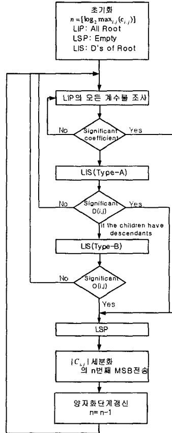
그림 2. SPIHT 알고리즘의 블록도
