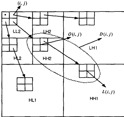
그림 1. Spatial Orientation Trees in SPIHT
