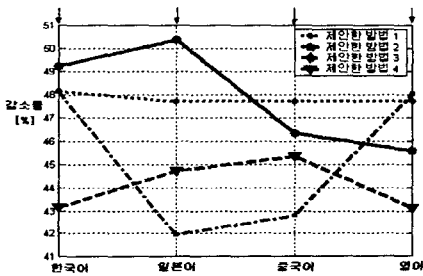
그림 6. (*, /) 계산량 감소율 비교(II)
