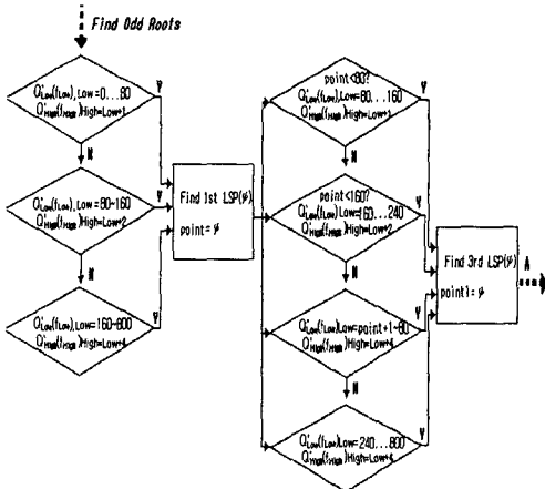
그림 4. 제안한 방법 4의 부분순서도
