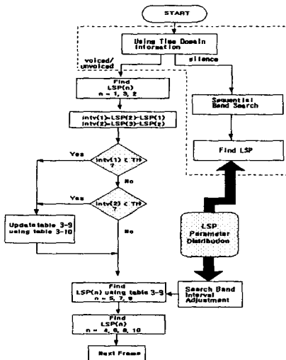
그림 3. 제안한 방법 3의 순서도
