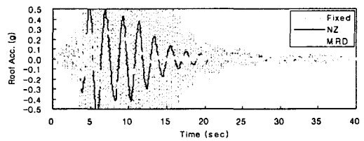
그림 12 Northridge 지진에 대한 Roof Acc. 비교
