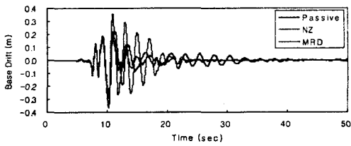
그림 8 Kobe 지진에 대한 Base Drift 비교
