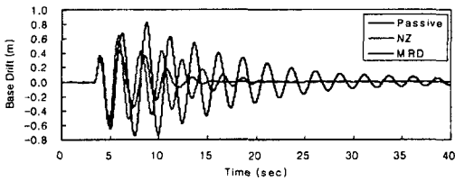
그림 11 Northridge 지진에 대한 Base Drift 비교
