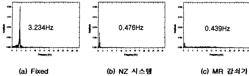
그림 13 Roof Acc. 에 대한 FFT 변환
