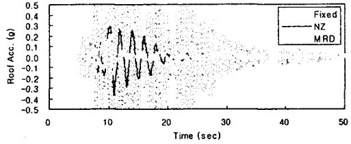
그림 9 Kobe 지진에 대한 Roof Acc. 비교
