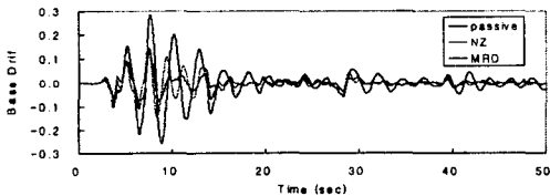
그림 5 El Centro 지진에 대한 Base Drift 비교
