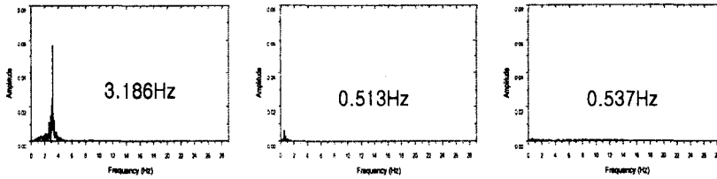
(a) Fixed (b) NZ 시스템 (c) MR 감쇠기
