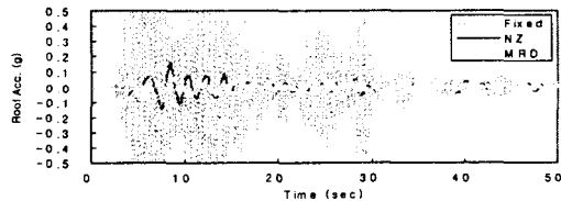
그림 6 El Centro 지진에 대한 Roof Acc. 비교
