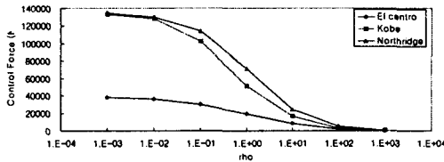
그림 2 \rho 값과 제어력의 관계
