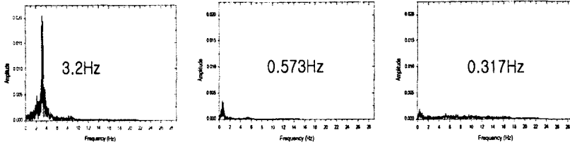
(a) Fixed (b) NZ 시스템 (c) MR 감쇠기
