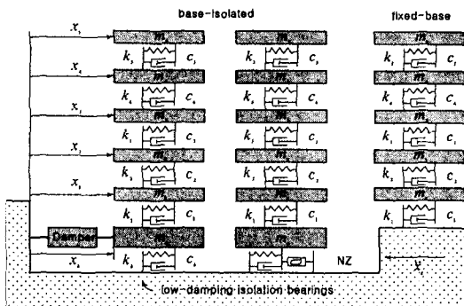
그림 1 수치해석 대상구조물
