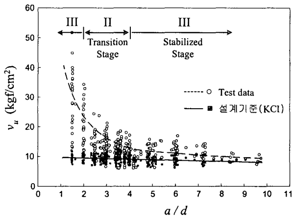
그림 2 전단보강철근이 없는 보의 전단강도
