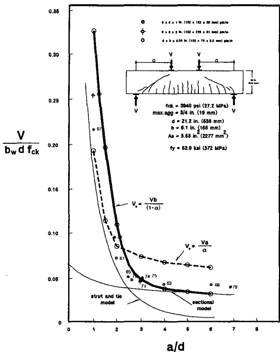
(a) Kani Test(1969) 3)
