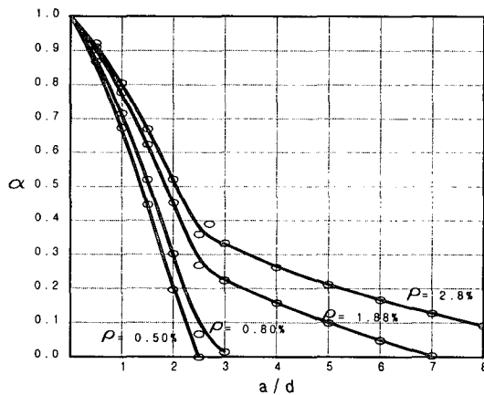
그림 3 a/d 변화에 따른 \alpha [kani 1969]
