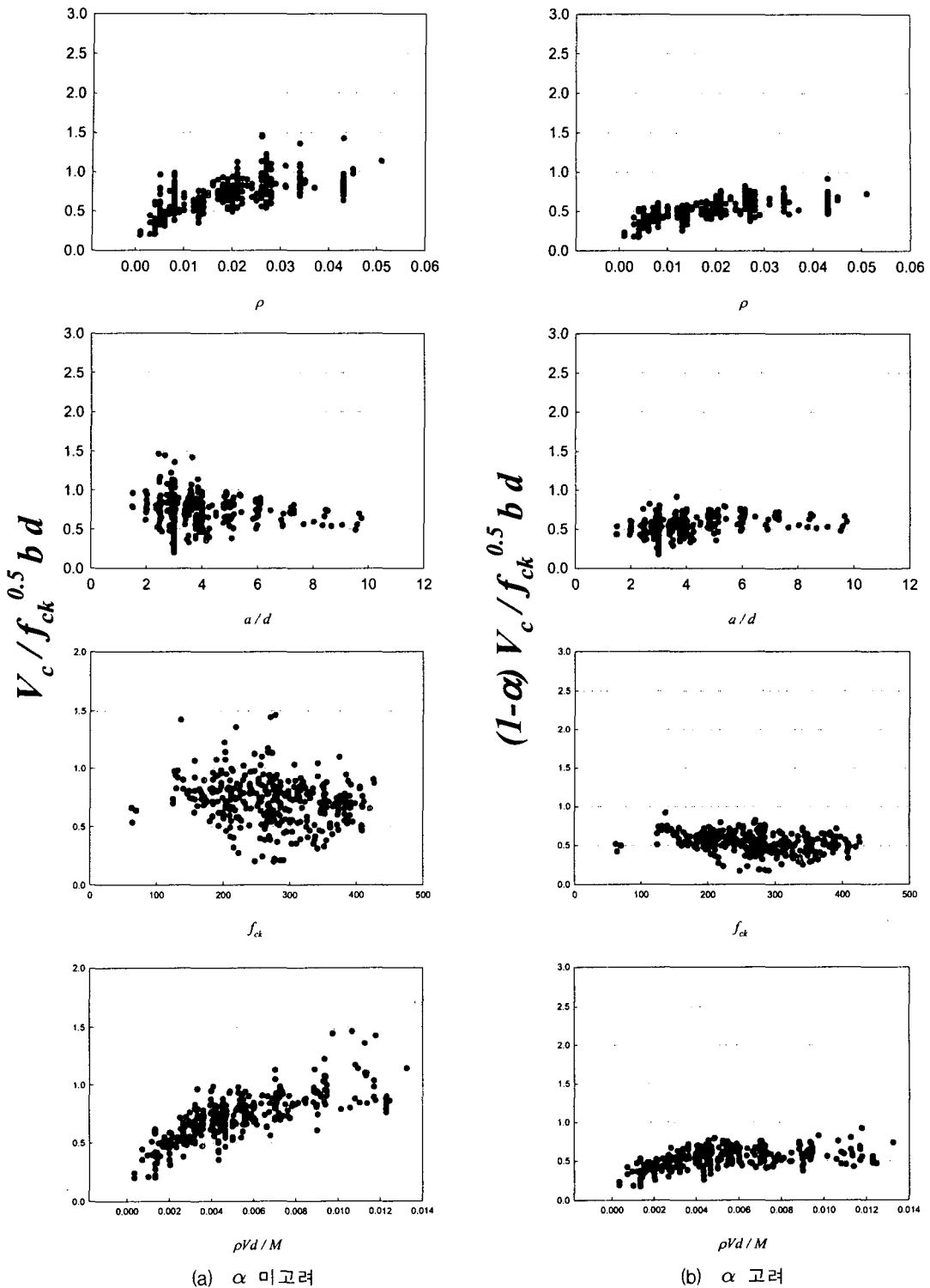
그림 5 내력상태계수 \alpha 를 통한 전단강도계수 상관
