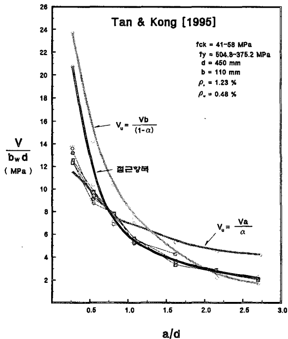
(b) Tan & Kong Test(1995) 6)
