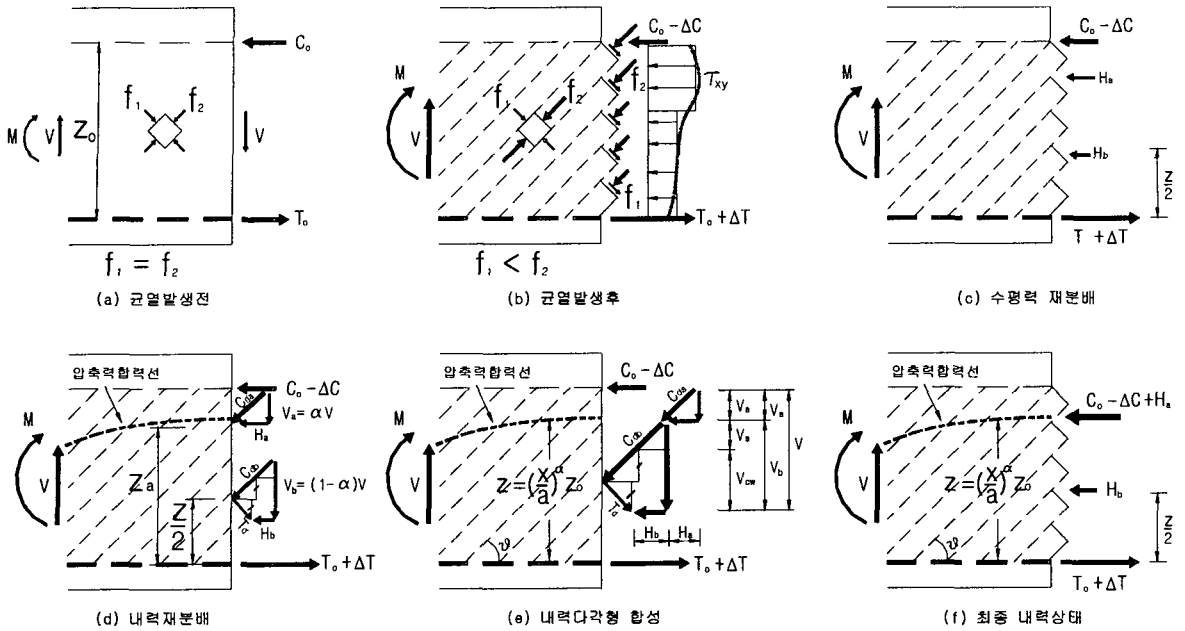
그림 1 균열전후 단면내력변화
