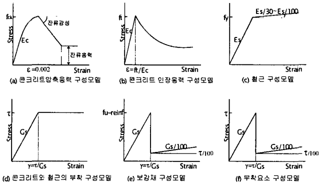
그림 4 사용요소의 재료비선형성
