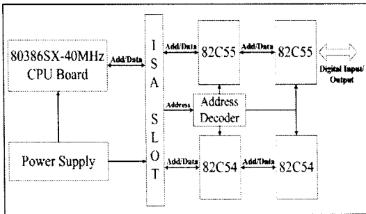
그림 3. 마킹 제어장치 블록선도
