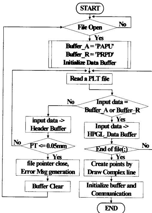
그림 5. CAD 데이터 추출 알고리즘
