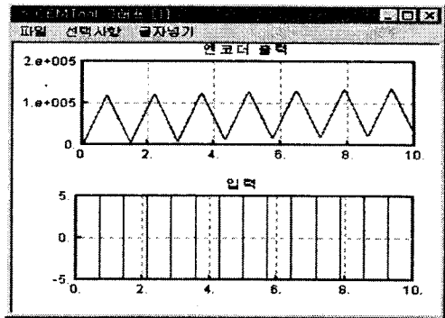
그림 5 시스템 식별을 위한 입출력 파형
