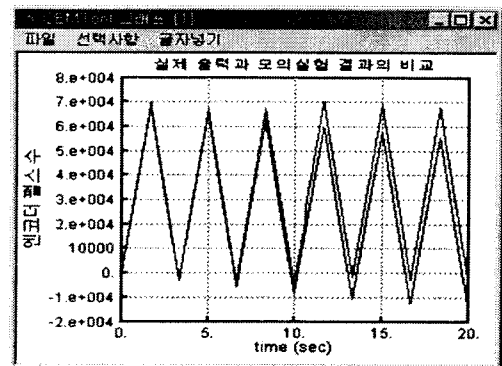
그림 6 실제 실험과 모의실험 결과비교
