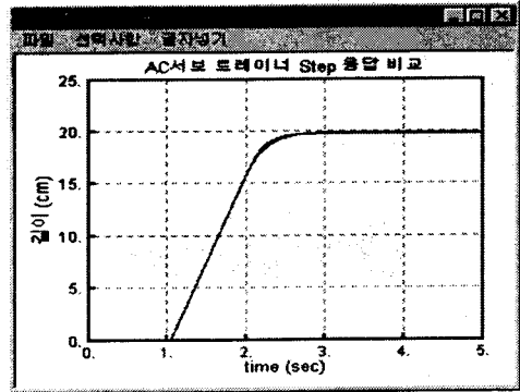
그림 10 모의실험과 실제실험결과 비교
