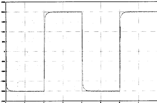
그림 8 속도 제어기 응답
