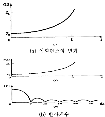
그림 1 테이퍼형 발룬의 특성
