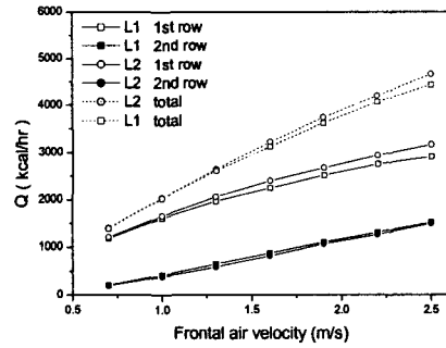
(a) louver fin
