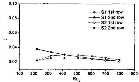
(b) slit fin
