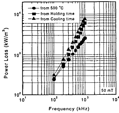
그림 5. 분위기 제어방법에 따른 전력손실
