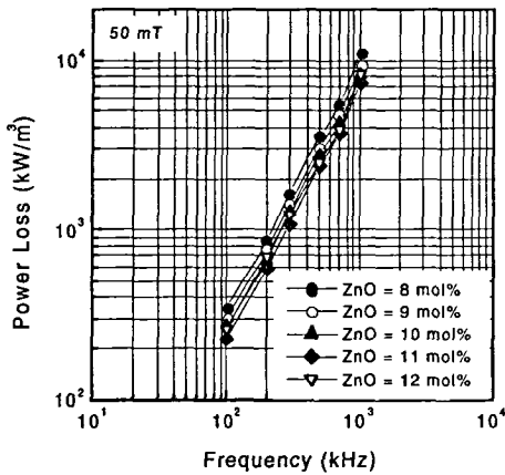
그림 3. 조성에 따른 전력손실 변화
