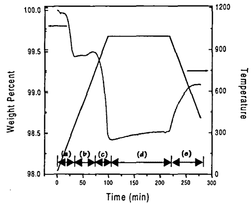
그림 1. Mn-Zn 페라이트의 열분석(TG) 결과
