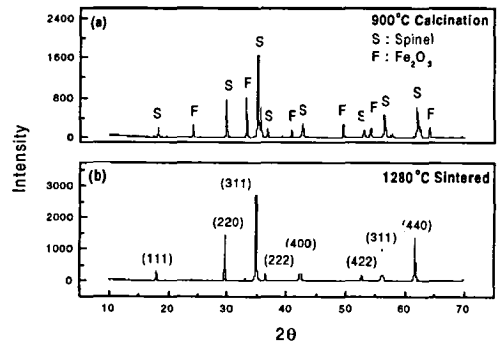
그림 2. X-ray 회절분석 결과
