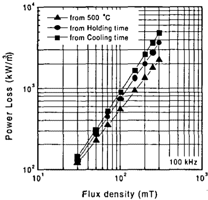
그림 6. 자속밀도에 따른 전력손실
