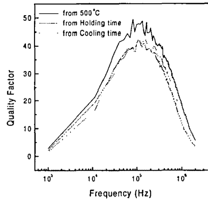
그림 8. 분위기 제어방법에 따른 품질계수
