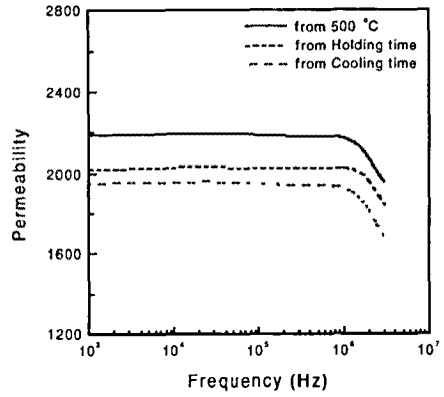
그림 7. 분위기 제어방법에 따른 투자율
