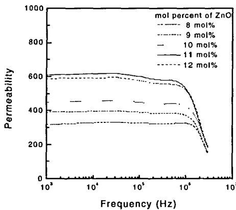
그림 4. 조성에 따른 투자율 변화
