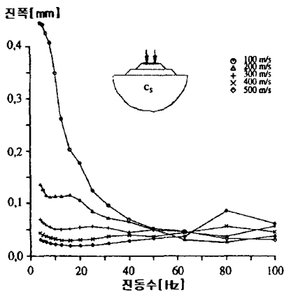
그림4. 지반특성에 따른 자갈케도의 수직변위변화
