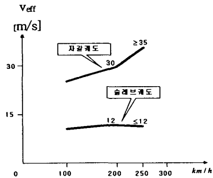
그림2. 열차속도에 따른 동적지반응답
