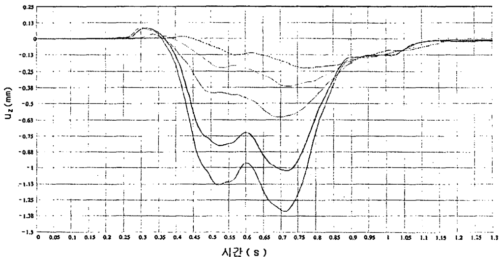
그림10. 시간에 대한 z방향 변위(궤도의 수직변위)
