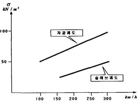
그림1. 열차속도에 따른 지반응력
