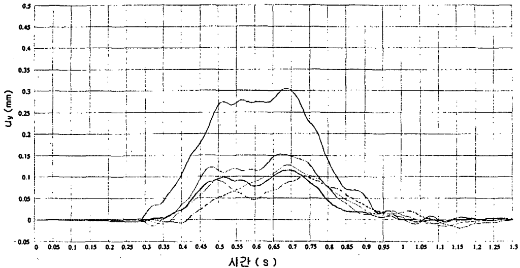
그림11. 시간에 대한 y 방향 변위(궤도의 횡방향)
