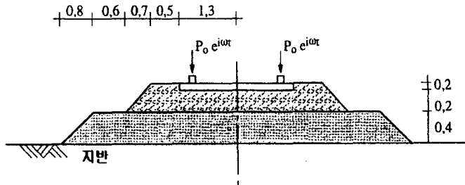
그림3. 기존자갈케도의 계산모델
