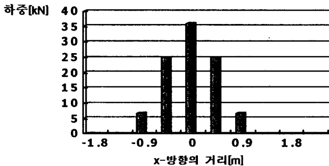
그림7. 해석을 위한 거리에 대한 열차의 이동하중분포
