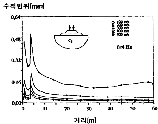
그림5. 지반특성에 따른 케도진동 및 파전달
