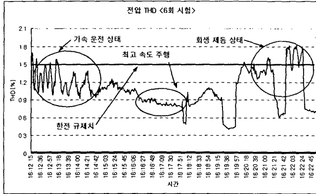
그림 13. KTX 주행상태에 따른 전압 왜형률
