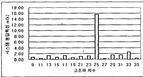
그림 9. 시스템 고조파응답특성 실측결과 (KPR=108km, 6MB(full), 전차선로=가압)
