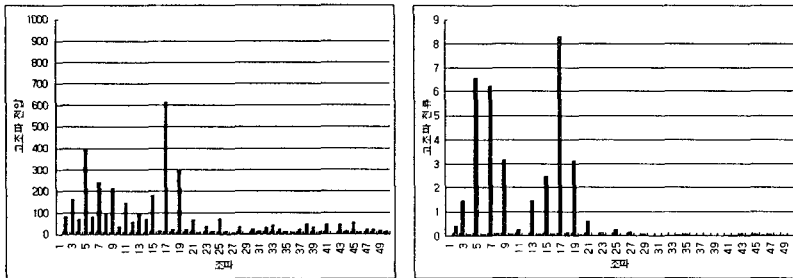
그림 10. 고조파 전압/전류 스펙트럼 (가속운전)
