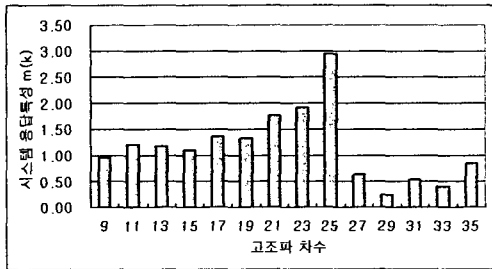
그림 7. 시스템 고조파응답특성 실측결과 (KPR=129km, 6MB(full), 전차선로=가압)
