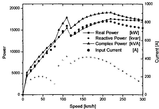
그림 1. KTX 차량의 전력 소비 특성
