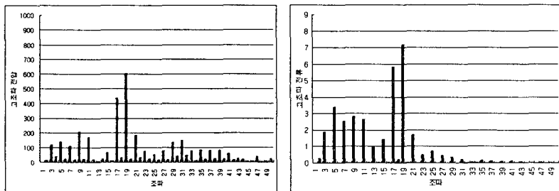
그림 12. 고조파 전압/전류 스펙트럼 (회생운전)
