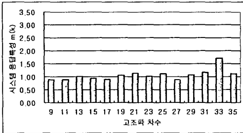
그림 6. 시스템 고조파응답특성 실측결과 (KPR=129km,, 6MB(full), 전차선로=차단)
