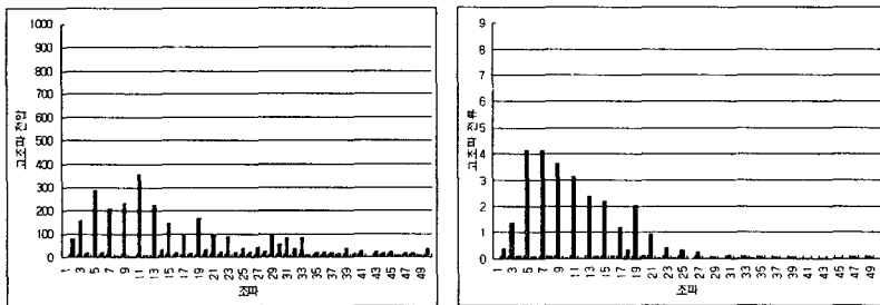
그림 11. 고조파 전압/전류 스펙트럼 (최고속도)
