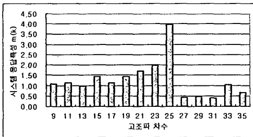
그림 8. 시스템 고조파응답특성 실측결과 (KPR=129km, 3MB(full), 전차선로=가압)
