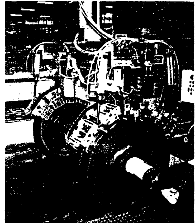
그림 3. Wheel test station AURA.
