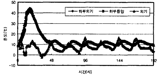
그림 3 수화열 측정실험
