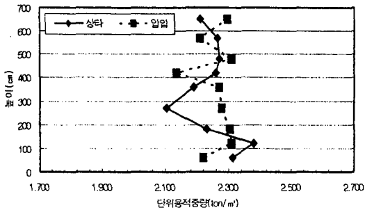
그림 5 코어 단위용적중량
