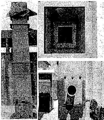
사진 1 강관의 외·내형 및 압입구
