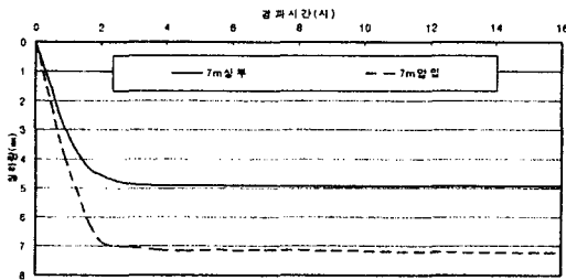
그림 2 침하량
