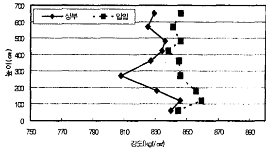
그림 6 코어 압축강도
