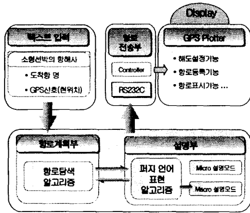
그림 1. 지능형 항해지원 시스템의 구성
