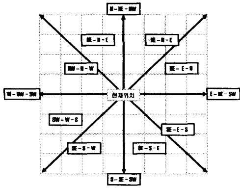
그림 3. 탐색 순서도
