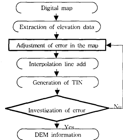
그림 1. 수치지도를 이용한 DEM의 생성과정
