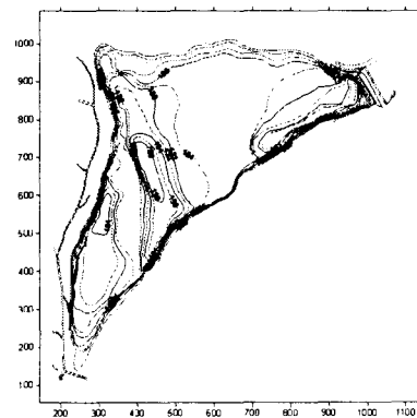
그림 4. base map
