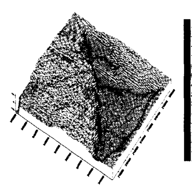
그림 7. wireframe
