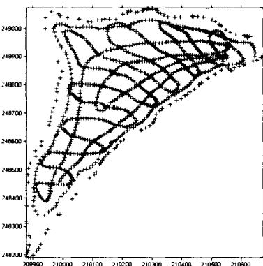
그림 5. post map
