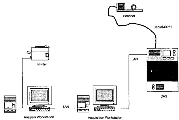
<그림 1> 자동초음파검사장비 시스템 구성도
