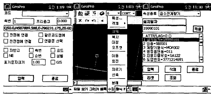
(a) 측량성과 (b) CAD 기능 (c) 속성편집기능
