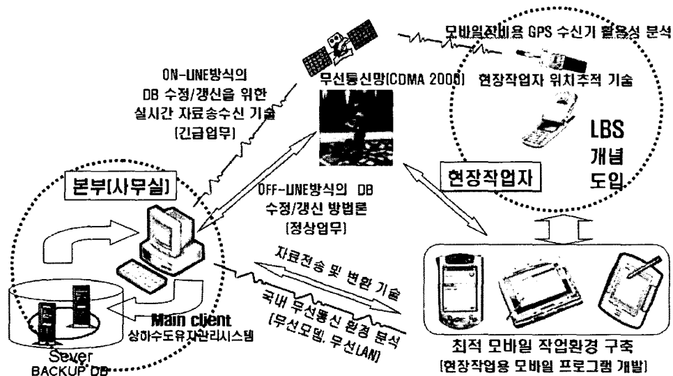
그림 1. 지하시설물 DB의 유지관리 방법론 개념도
