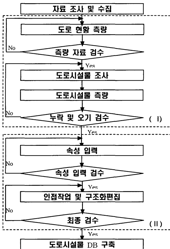
그림 1. 도로시설물 DB구축 과정
