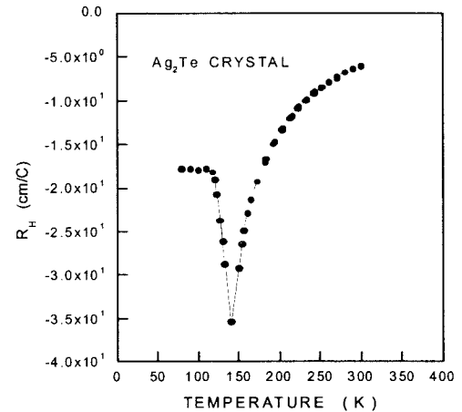
그림 5. Ag_2Te 단결정에서 Hall 계수의 온도의존성. Fig. 5. Temperature dependence of Hall coefficient in Ag_2Te single crystal.
