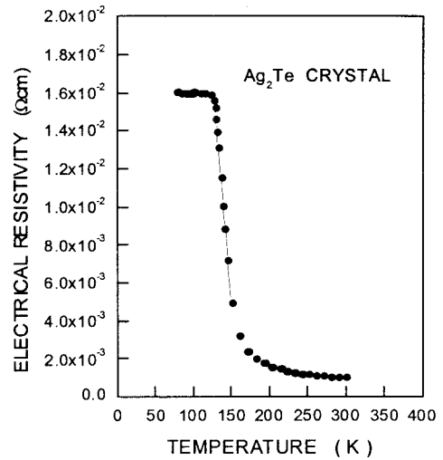
그림 4. Ag_2Te 단결정에서 비저항의 온도의존성. Fig. 4. Temperature dependence of electrical resistivity in Ag_2Te single crystal.
