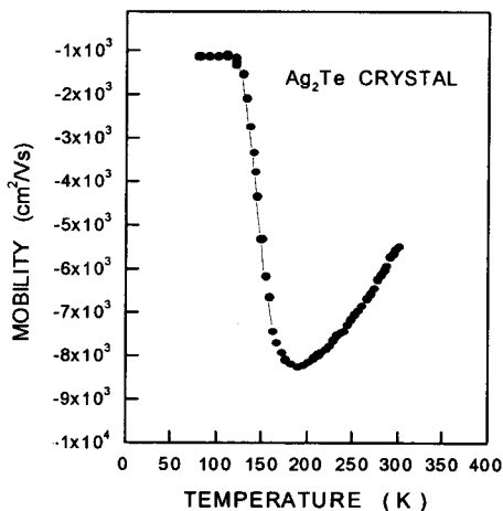
그림 7. Ag 2 Te 단결정에서 전자 이동도의 온도의존성. Fig. 7. Temperature dependence of electron mobility in Ag 2 Te single crystal.
