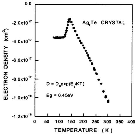
그림 6. Ag 2 Te 단결정에서 캐리어 농도의 온도의존성. Fig. 6. Temperature dependence of carrier concentration in Ag 2 Te single crystal.
