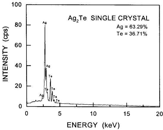
그림 2. Ag_2Te 단결정의 성분분석 Fig. 2. EDX pattern of sintered Ag_2Te single crystal
