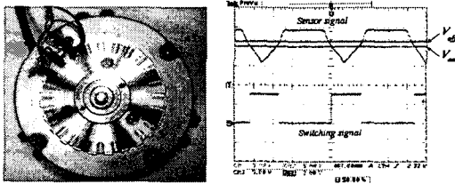
그림 5. SRM에 장착된 엔코더와 엔코더의 출력파형 Fig 5. Prototype encoder and output signals
