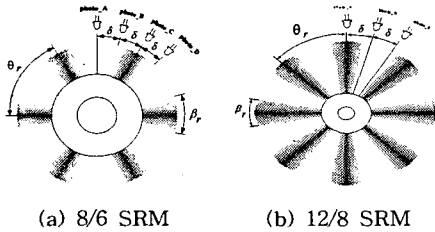
그림 2. 제안된 아날로그 엔코더용의 디스크판 Fig. 2. Disk plate proposed for analog encoder
