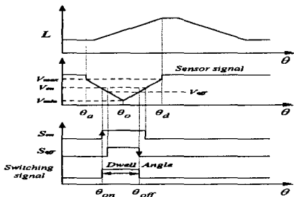
그림 3. 상스위칭 각 독립제어원리 Fig. 3. Principle of switching angle independent control
