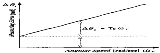
그림 1. 회전자 속도에 따른 회전자 위치의 측정오차 Fig. 1. Measuring error of rotor position according to rotor speed
