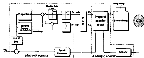
그림 4. 제어 시스템의 블록도 Fig. 4. Block diagram of the control system
