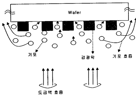
(a) 분수형 도금장치의 Face-down형 링
