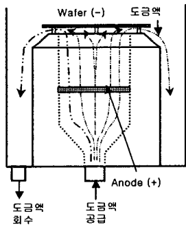
그림 2. 분수형 도금장비 Fig.2 Fountain plating system
