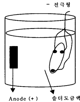
그림 3. 경사형 전극링 도금장치 Fig 3. Tilted electrode ring plating system
