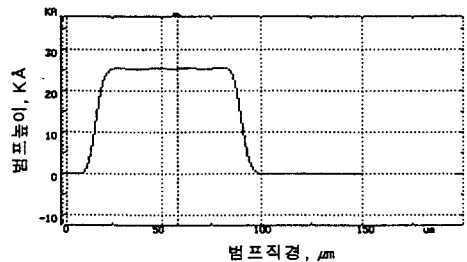
그림 7. 경사진 링구조의 도금장치에서 형성된 솔더박막의 두께 Fig. 7 Thickness of solder layer formed by the tilted electrode ring plating system
