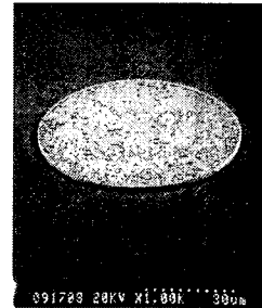
그림 6. 경사진 링구조의 도금장치에서 형성된 솔더 박막 Fig. 6 Solder layer formed by the tilted electrode ring plating system
