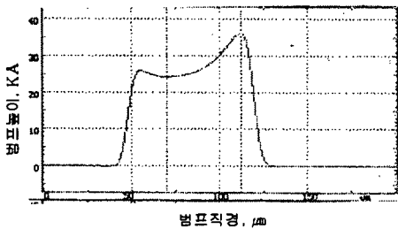
그림 5. 분수형 도금장비를 사용하여 형성된 솔더 박막의 두께 Fig. 5 Thickness of solder layer formed by fountain plating system
