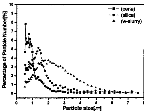
그림 4. slurry의 입도분석. Fig. 4 particle size analysis of different slurry.
