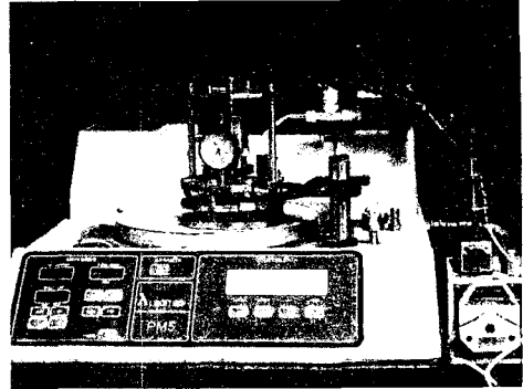
그림 1. CMP 장비.
