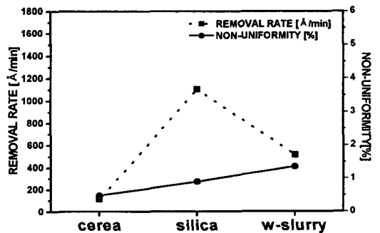
그림 2. 슬러리 종류에 따른 연마율과 비균일도.
