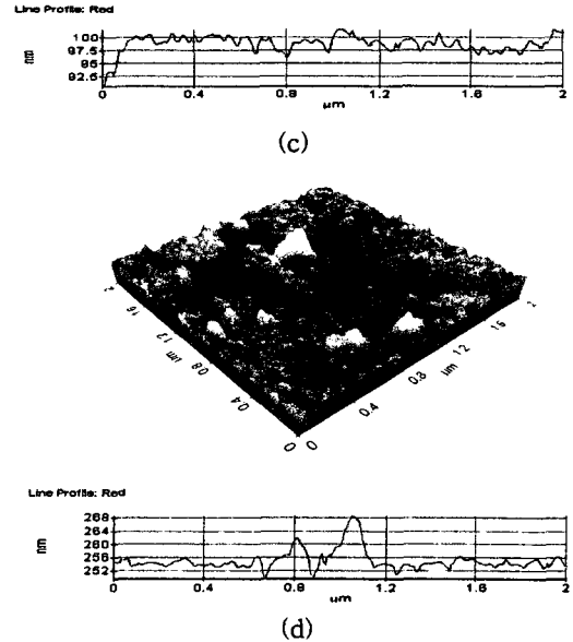
그림 3. 슬러리 종류에 따른 AFM 형상과 거칠기 (a)CMP전 (b)실리카 (c)세리아 (d)텅스텐. Fig. 3 AFM image of different slurry (a)pre-CMP (b)Silica (c)Ceria (d)Tungsten.
