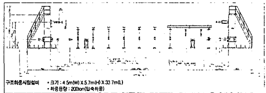
그림 12. 하이브리드 복합재 차체 구조시험 장비
