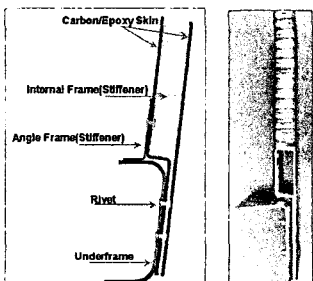
그림 11. 복합재 차체와 금속재 언더프레임간의 체결
