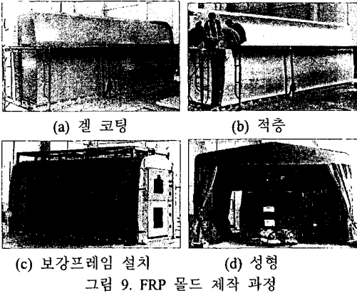
그림 9. FRP 몰드 제작 과정
