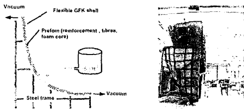
그림 3. Vacuum Infusion에 의한 전두부 제작 공정
