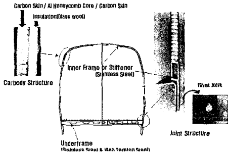
그림 1. TTX 하이브리드 복합재 차체 단면 구성도
