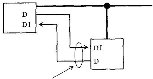
Flag감시용 입출 그림 4 Flag감시방식
