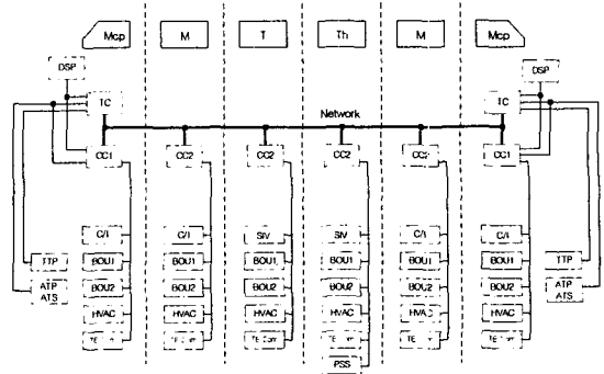
그림 3 TMS 인터페이스 구성도
