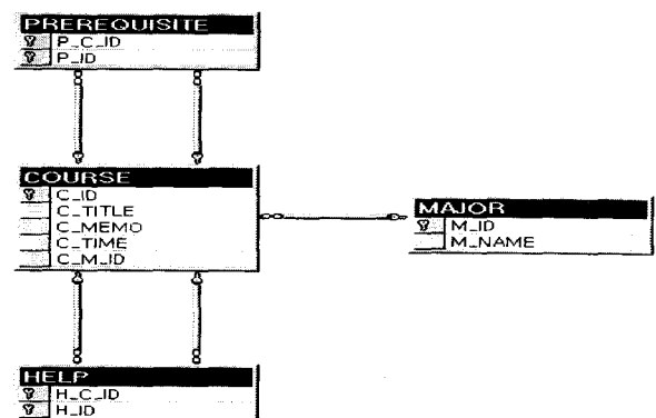
〈그림 2〉 E-R 다이어그램
