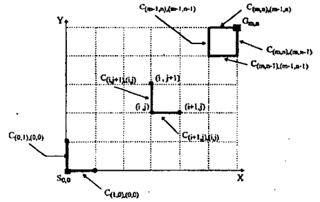
그림 4 동적계획법을 위한 2차원 격자 경로 Fig. 4 2-Dimension Grid Path for Dynamic Programming
