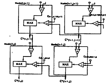
그림 5 제안방식 신경회로망을 이용한 동적계획법의 구현
