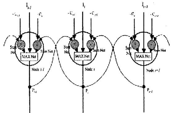
그림 3. 제안한 신경망의 1차원구조와 노드구조 Fig. 3. 1-Dimension Node of Proposed LIPN
