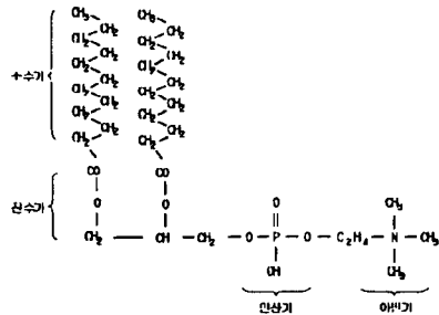
(b) DMPC
