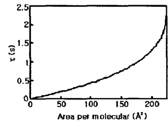
(b) DMPC
