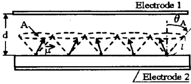
그림 1. 수면위의 분자모델
