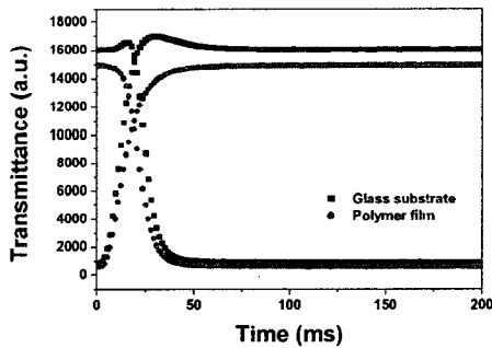
그림 6. 고분자 및 유리기판을 이용한 경우 폴리이미드 표면에서의 응답 특성.
