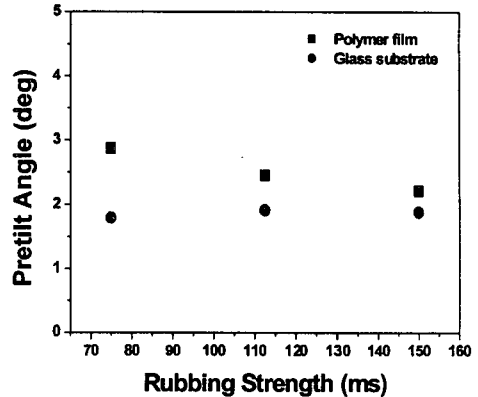
그림 4. 두가지 종류의 기판을 이용한 폴리이미드 표면에서의 러빙강도에 따른 네마틱액정의 틸트각.
