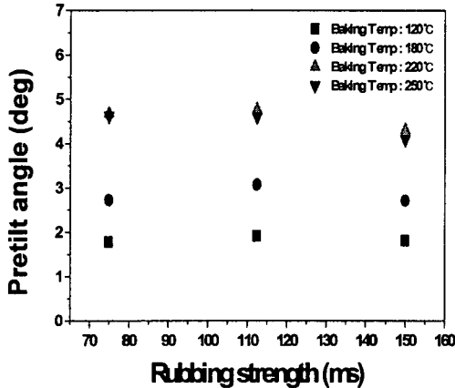
그림 3. 유리기판을 이용하여 폴리이미드 표면에서의 소성 온도에 따른 네마틱 액정의 프리틸트각의 발생.
