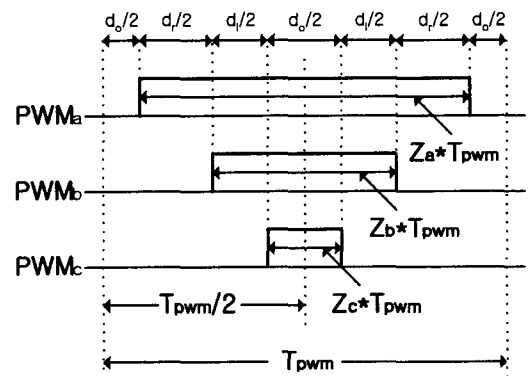
그림 3.2 PWM 인버터 듀티사이클 배열
