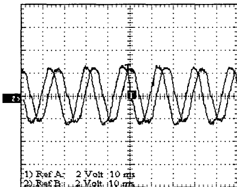
그림 4.3 인버터 상전류
