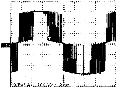
그림 4.2 인버터 선간전압
