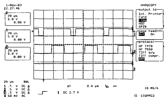
그림 4.1 인버터 게이트 신호
