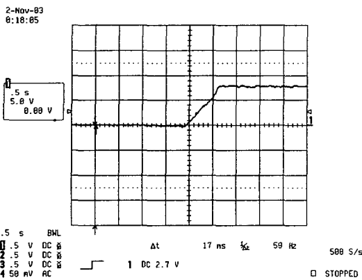
그림 4.4 무 부하시의 정격 속도 응답
