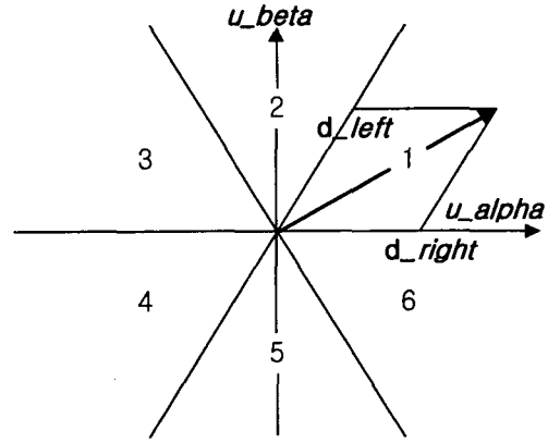
그림 3.1 공간벡터 변조 PWM
