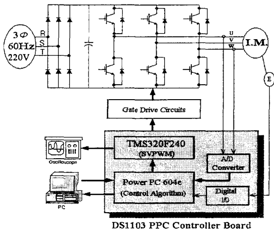
그림 3.3 시스템 구성도
