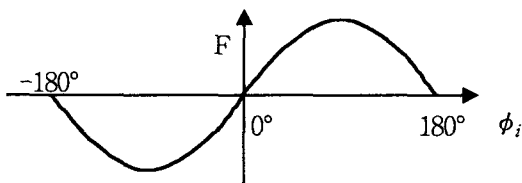
그림 2 전기각도로 나타낸 초기 자극위치에 대한 추력
