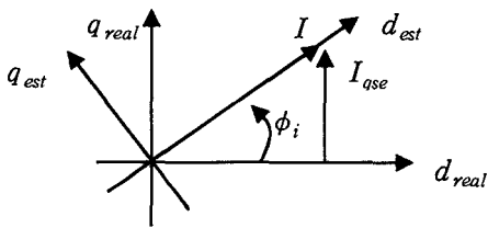
그림 1 동기좌표계상의 초기 자극위치
