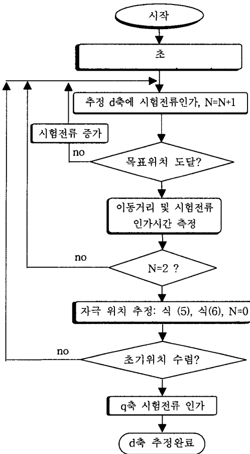
그림 3 초기 자극위치 추정 순서도
