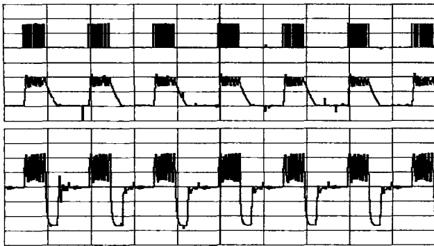
그림 11 측정된 게이트 신호와 상전압 및 상전류 파형 Fig. 11 Measured gate signal, phase voltage and current wave at 2,000[rpm]
