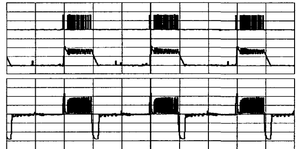
(X=0.5ms/div, Y=2.5V/div, 2A/div, 150V/div) 그림 9 측정된 게이트 신호와 상전압 및 상전류 파형 Fig. 9 Measured gate signal, phase voltage and current wave at 1,000[rpm]
