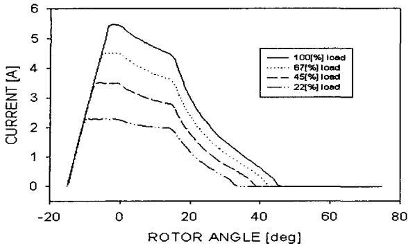
(a) 전류파형
