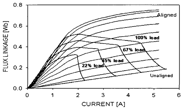
(b) 쇄교자속
