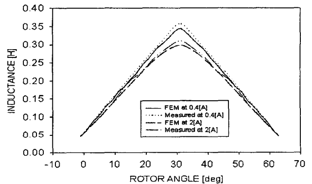
그림 5 인덕턴스 측정치와 해석치 비교 Fig. 5 Comparison of measured and analytical inductance
