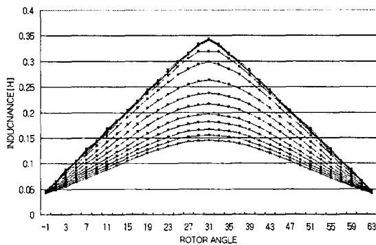
그림 3 회전에 따른 인덕턴스 변화 Fig. 3 Various inductance with rotor angle
