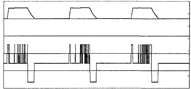
그림 8 시뮬레이션에 의한 전압과 전류파형 Fig. 8 Simulated phase voltage and current wave
