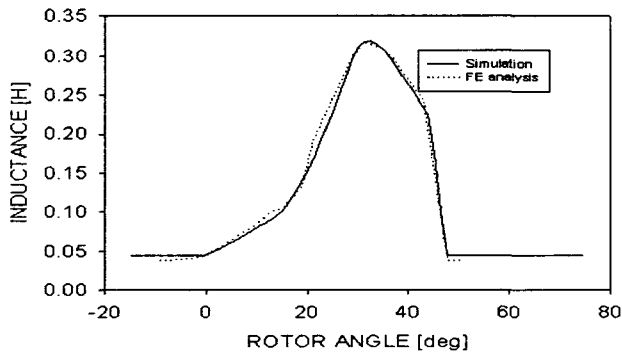
그림 7 인덕턴스 파형 비교 Fig. 7 Comparison of inductance profile
