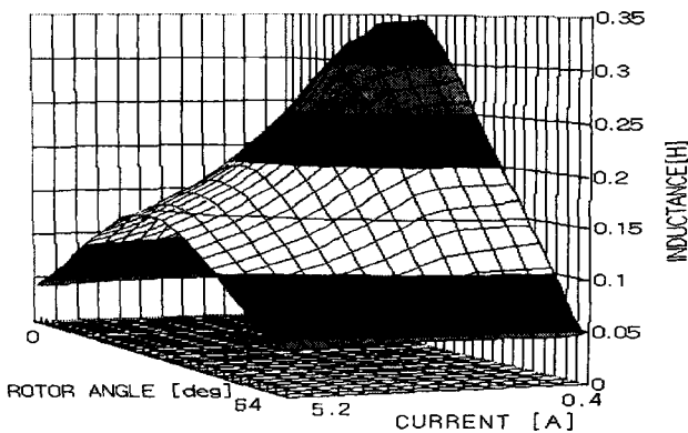
그림 2 회전각과 전류변화에 따른 인덕턴스 변화 Fig. 2 Various inductance with varied rotor angle and current
