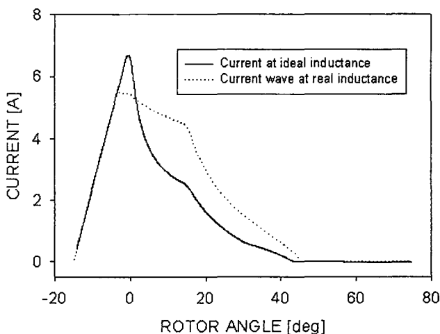
그림 12 이상적인 인덕턴스 적용시와 실제 인덕턴스 적용시 전류 파형 변화 비교
