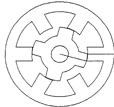
그림 1 6/4극 SRM의 구조 Fig. 1 Structure of 6/4 SRM
