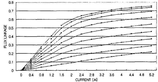
그림 4 회전각과 전류에 따른 쇠교자속 Fig. 4 Flux linkage versus rotor angle and current
