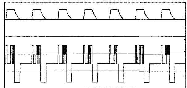
그림 10 시뮬레이션에 의한 전압과 전류파형 Fig. 10 Simulated phase voltage and current wave
