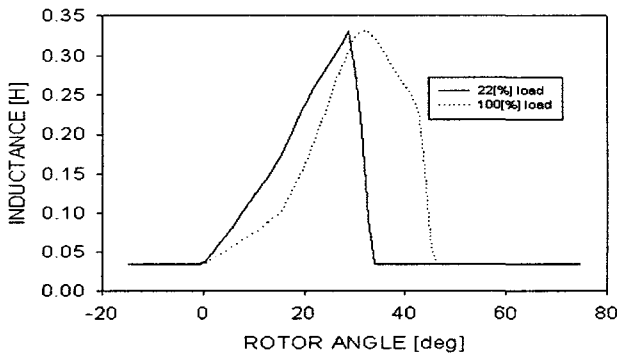
(c) 인덕턴스 파형
