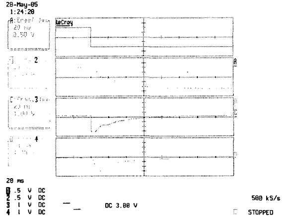
그림 8. 감속시 스텝응답(400→200RPM)
