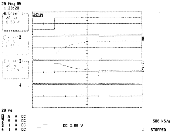
그림 7. 가속시 스텝응답(200→400RPM)
