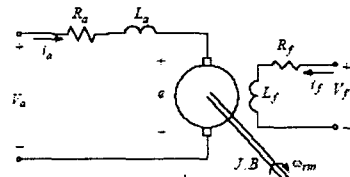
그림 1. 직류전동기
