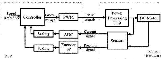
그림 3. 전체 시스템 구성도
