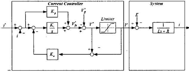
그림 2. PI 전류제어기
