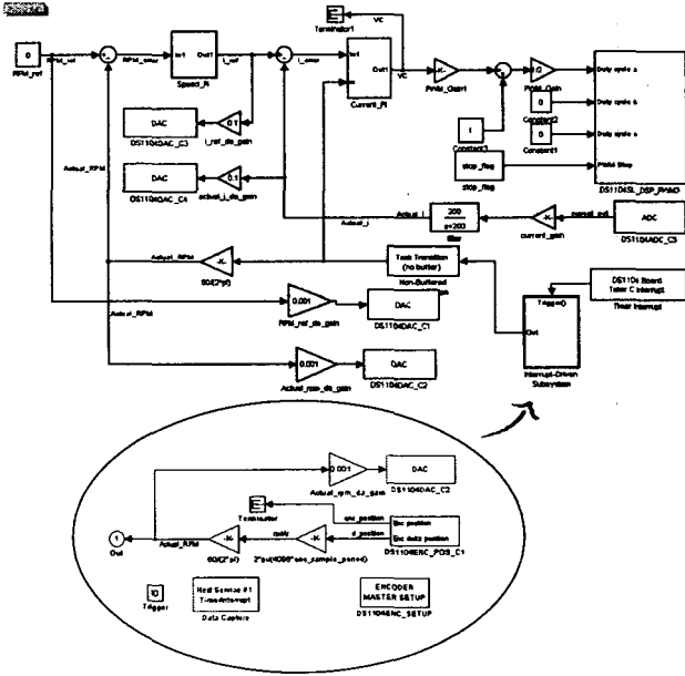
그림 6. 제어블록
