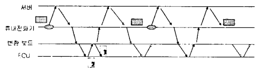
(b) 제안하는 방식의 통신 sequence
