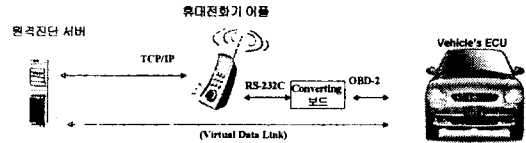
그림 2. 제안하는 차량진단 시스템의 구성
