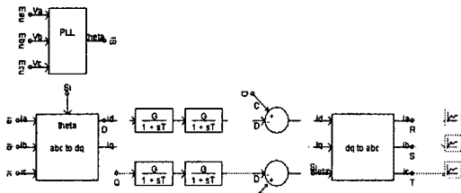
그림 4 고조파전류 보상위한 Active Filter 제어 블럭 다이어그램
