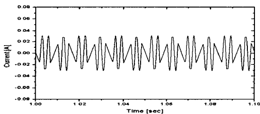
그림 5 Active Filter 통해 발생된 고조파 성분 전류 파형
