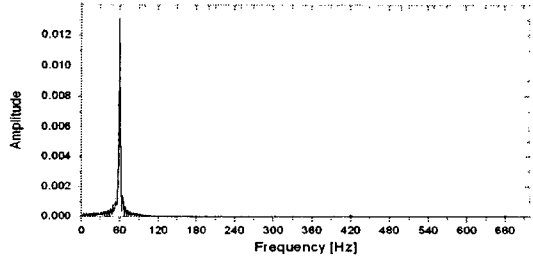
그림 7 고조파 전류성분이 보상된 계통전류의 결과
