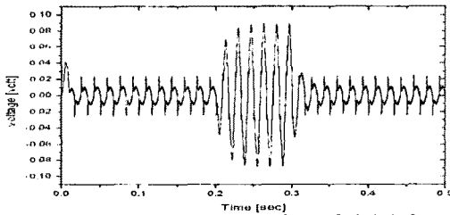
그림 11 컨버터를 통해 나온 전압보상전압파형( V_2 )
