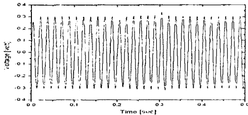
그림 12 전압강하 보상후의 계통전압 파형
