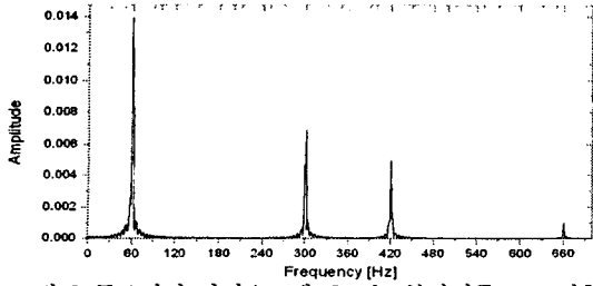
그림 3 풀브릿지 다이오드에 흐르는 부하전류FFT 변환
