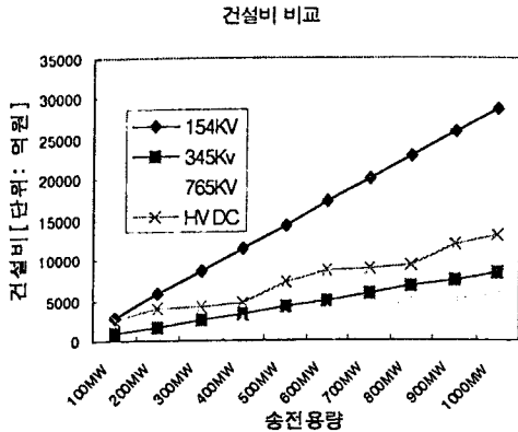
그림 2. 송전용량에 따른 송전선 건설비 비교(100Km)
