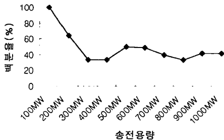
그림 3. 송전용량의 증가에 따른 건설비차 비율(%)
