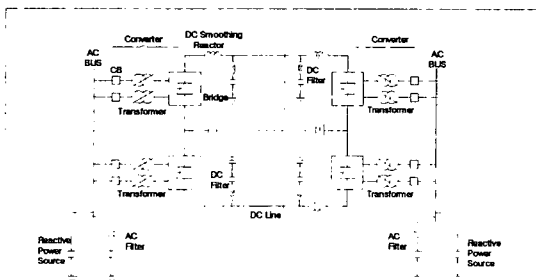
그림 1. 양극 HVDC 시스템의 주요 구성요소의 구성도
