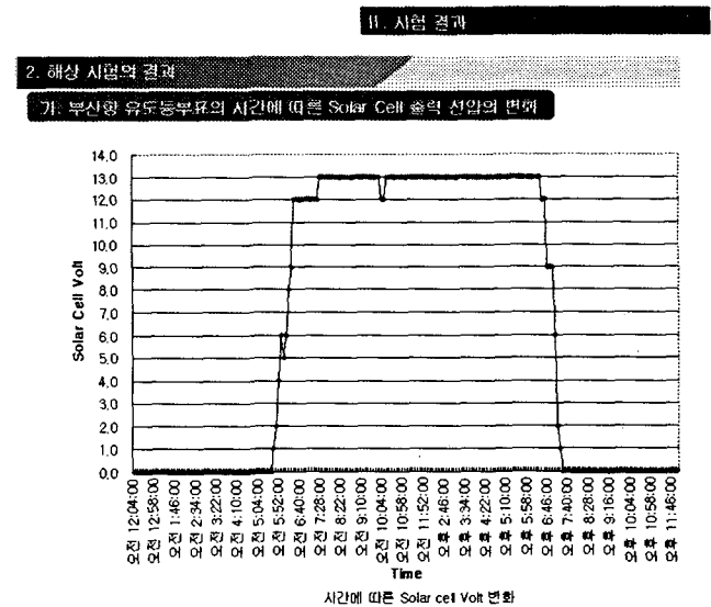
<그림 3-1> 부산항유도등부표의 Solar Cell 전압변화
