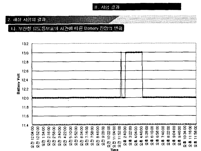
<그림 3-2> 부산항유도등부표의 축전지 전압변화
