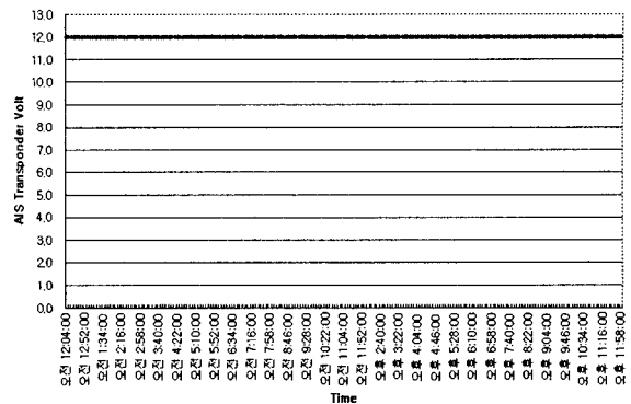
<그림 3-5> 부산항유도등표의 AIS Transponder의 전압변화
