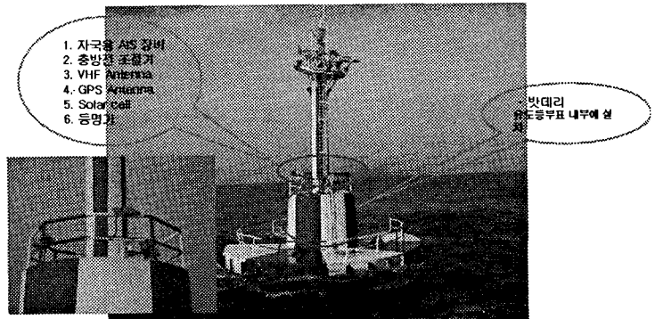
<그림 2-6> 부산항유도등부표에 장비의 설치현황
