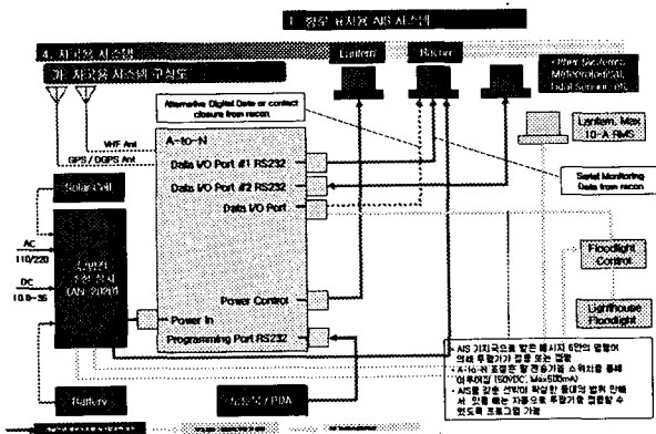
<그림 2-5> 자국 장비의 구성도
