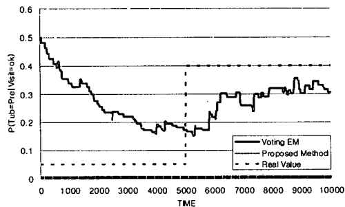
그림 4. 시간에 따른 비교 (학습률 4%, 데이터 손실률 0%)
