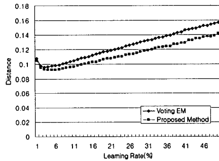
그림 3. 학습률에 따른 실제 해와의 거리
