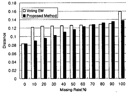
그림 2. 데이터 손실률에 따른 실제 해와의 거리
