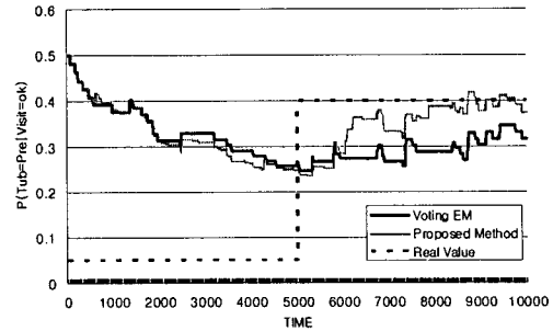
그림 5. 시간에 따른 비교 (학습률 4%, 데이터 손실률 50%)
