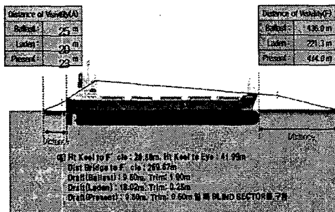
Fig. 11 선박의 맹목구간
