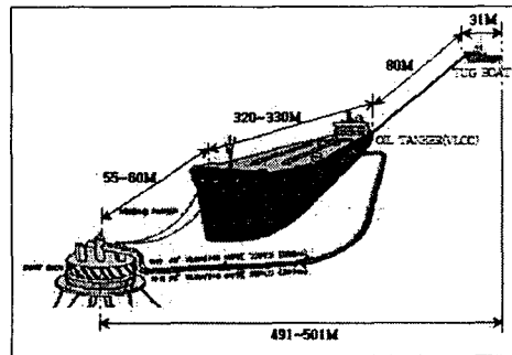
Fig. 3 원유부이 제한구역 기준
