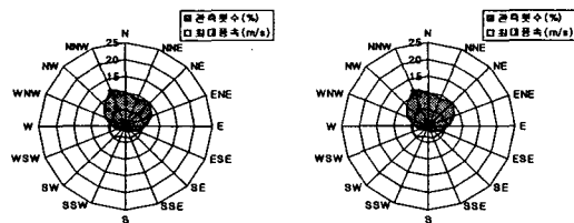
Fig. 6 가을철 및 겨울철 풍향별 풍속 및 관측횟수
