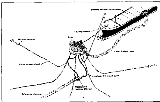
Fig. 1 Single Point Mooring의 배치도
