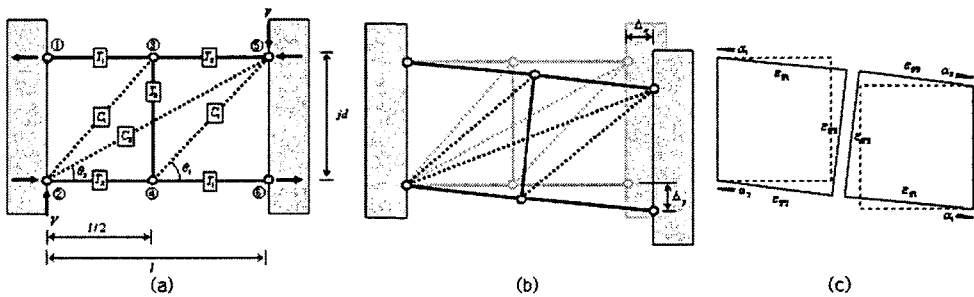
그림 2. (a) 기호의 정의 (b) 연결보의 변형 (c) 타이의 인장변형과 경사각
