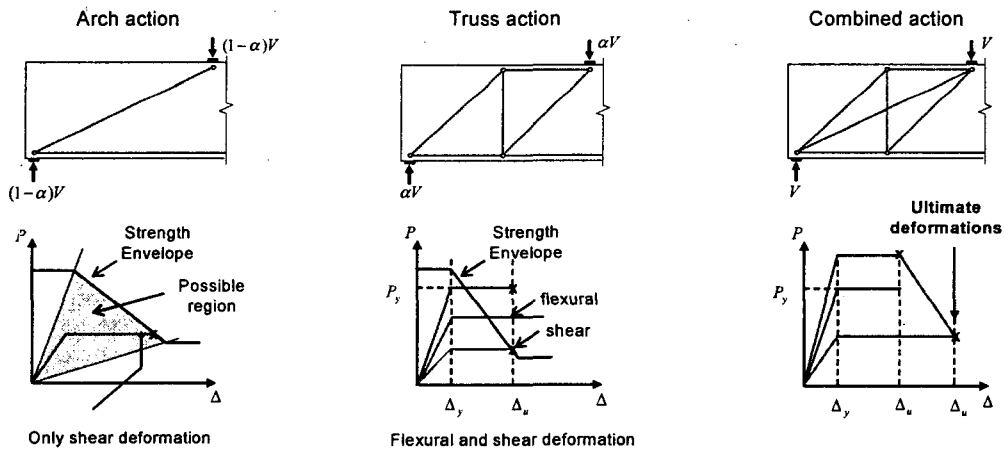
그림 1. (a) 아치작용 (b) 트러스 작용 (c) 조합작용
