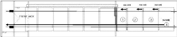
그림22. 1차견인
