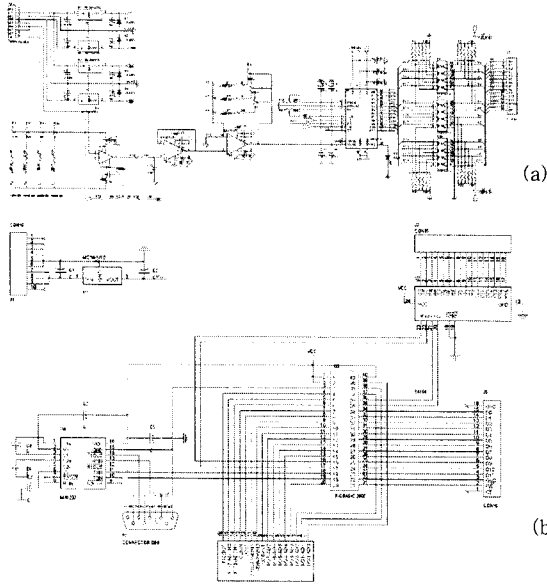
그림 2. (a) 로드셀 센서 신호 증폭, 필터링, A/D 변환 회로도. (b) 16 채널 전체 제어 회로도
