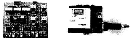
그림 3. (a) 1채널 센서 신호 증폭기, 필터링, A/D 변환기 (b) PIC16F877 마이크로컨트롤러를 내장한 PBM-R5 모듈, 디코더, Bluetooth 송수신 모듈
