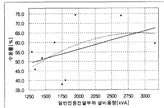
그림 3. 일반전등전열 부하의 수용률 적용 실태 및 회귀 모형식
