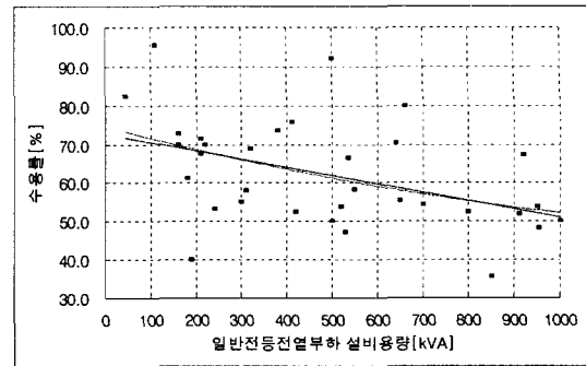
그림 2. 일반전등전열 부하의 수용률 적용 실태 및 회귀 모형식
