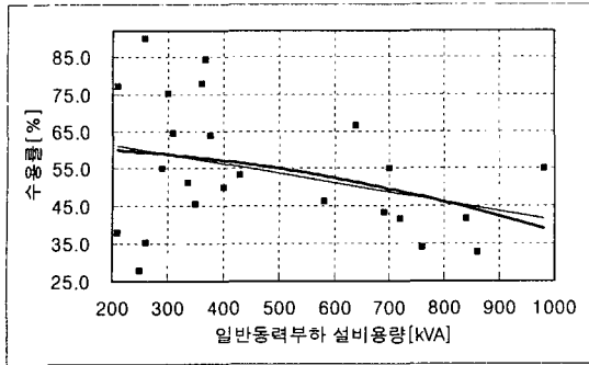
그림 5. 일반동력부하의 수용률 적용 실태 및 회귀 모형식
