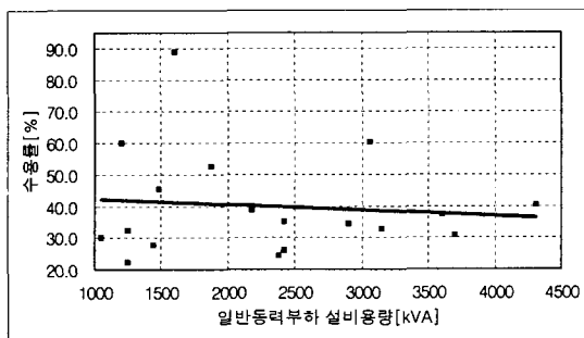
그림 6. 일반동력부하의 수용률 적용 실태 및 회귀 모형식
