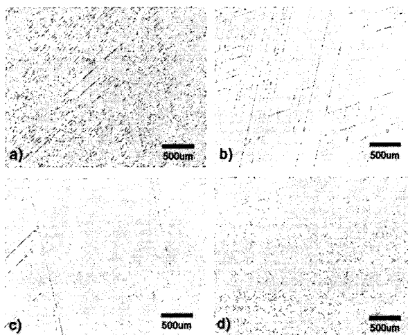
그림 1. AlN 완충층 두께에 따른 GaN 박막의 표면 사진.
