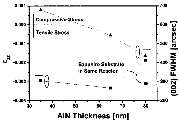
그림 3. AlN 완충층 두께에 따른 GaN 박막의 out-plane 응력과 (002) FWHM.
