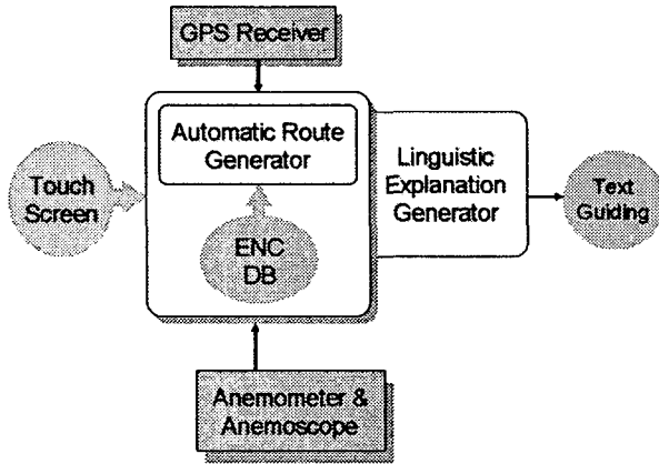
그림 4. INGS의 블록선도
