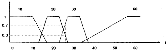
그림 12. 도달시간 데이터의 언어레이블 표현
