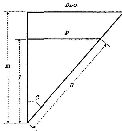
그림 7. 점장위도항법
