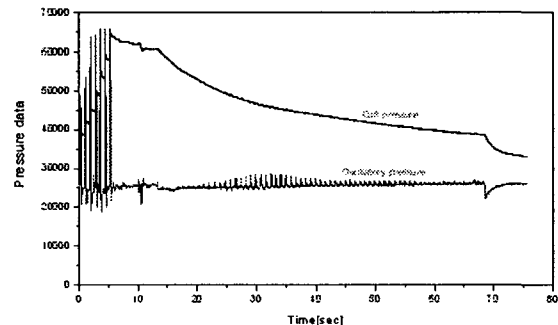
그림 6. Cuff내 압력변화신호(상)와 박동신호(하)의 예.
