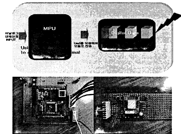
그림 3. 송신시스템의 구성
