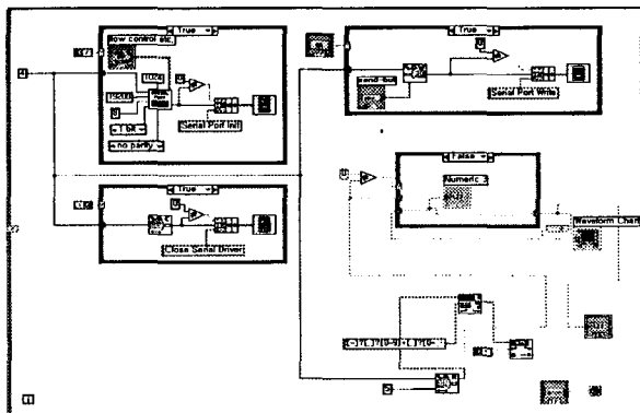
그림 7. Labview의 블록 다이어그램
