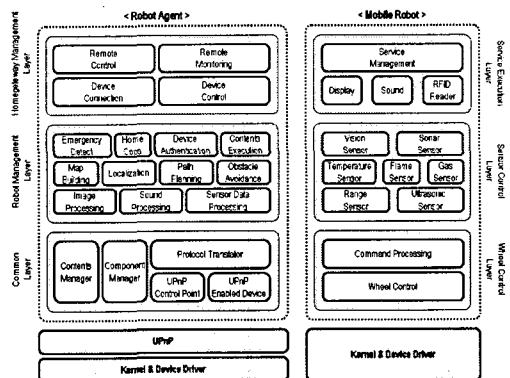
▶▶ 그림 3. 로봇 에이전트 아키텍처
