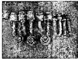
Fig 6. 볼트 파손 사진
